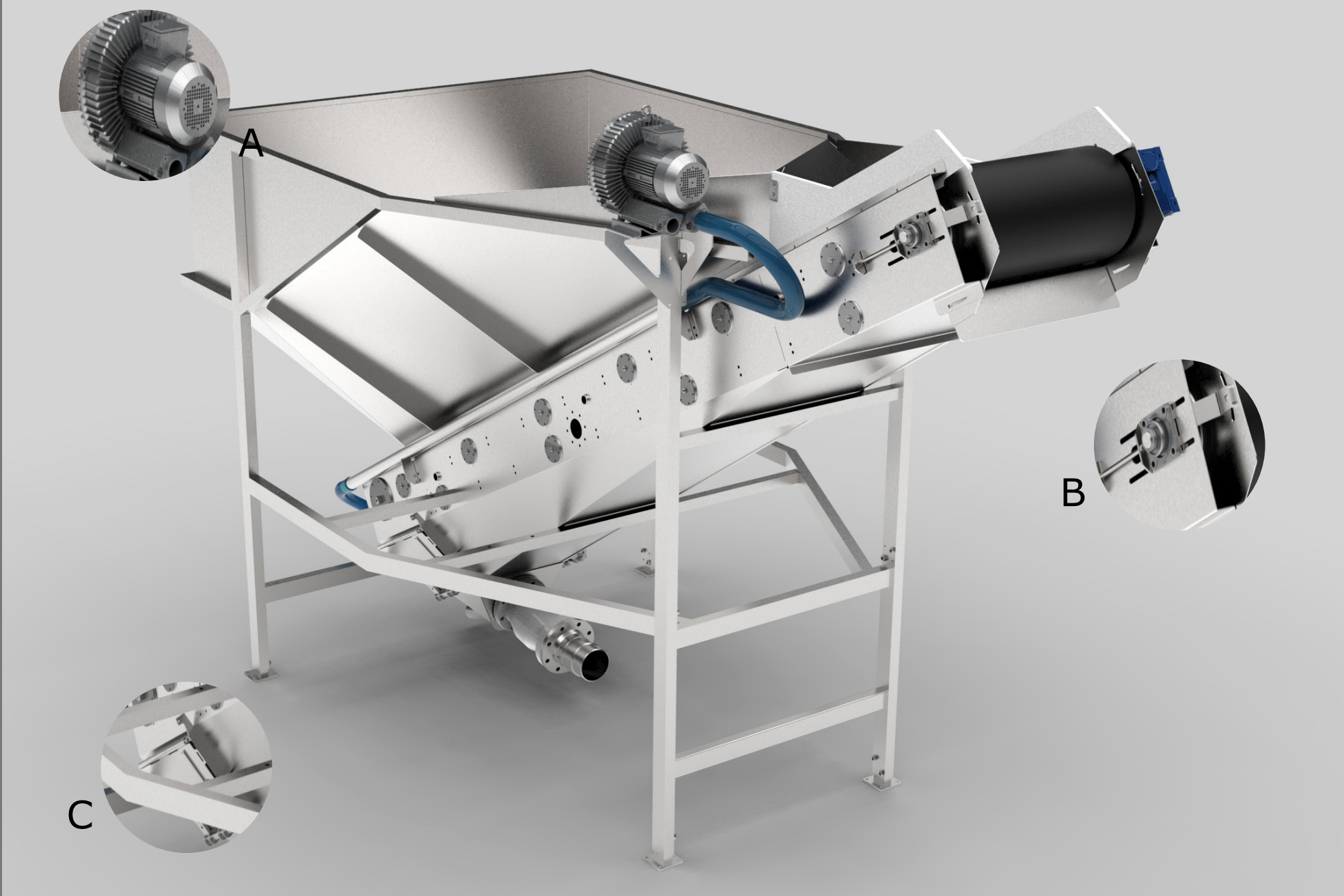
C Inspection door
